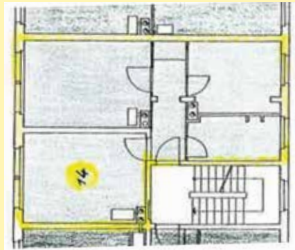
Abb.: Wohnungsgrundriss
